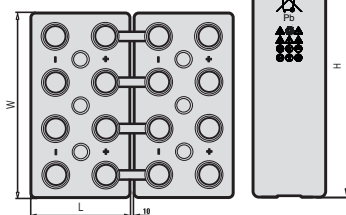
Fig. F Type OPzV
